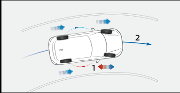
Control activo en curva (AYC)
